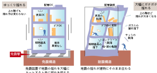
免震構造と耐震構造の違い
